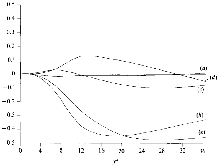
FIGURE 3. Spatial dependence of terms in Reynolds stress decomposition (3): (a) \overline{u_b v_a} ; (b) gradient term; (c) \Phi_1 ; (d) \Phi_2 ; (e) \overline{wv} .
